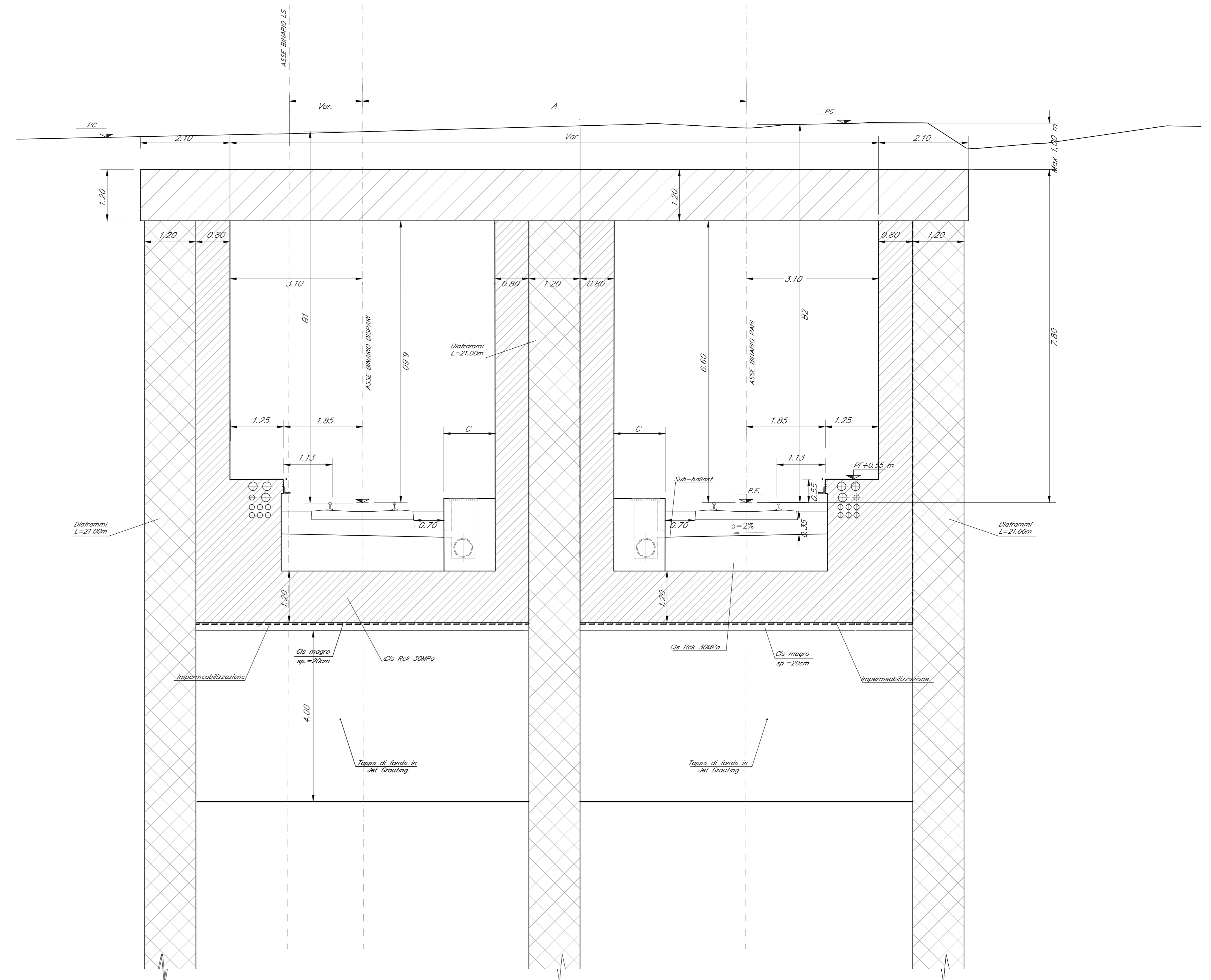
Sezione Tipo 3
