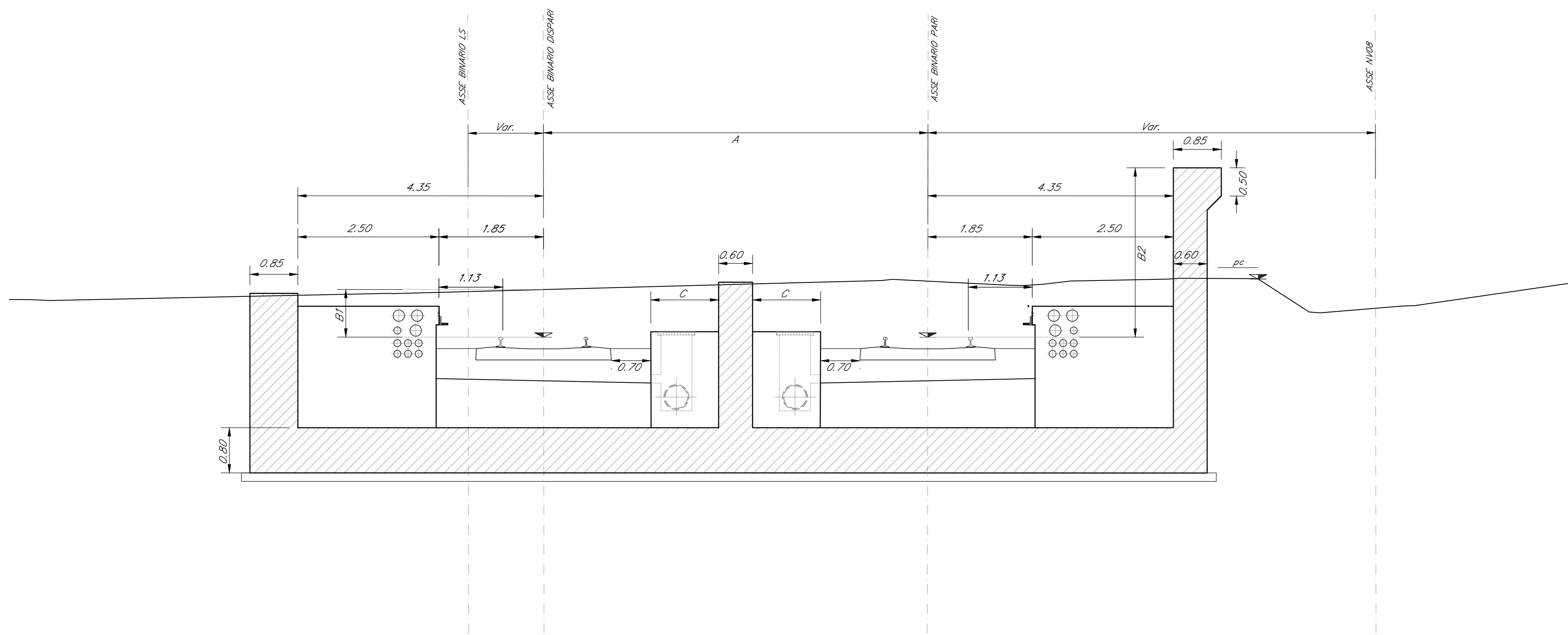
Sezione Tipo 4.1
