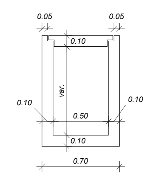
Dettaglio "2" - Canaletta idraulica
