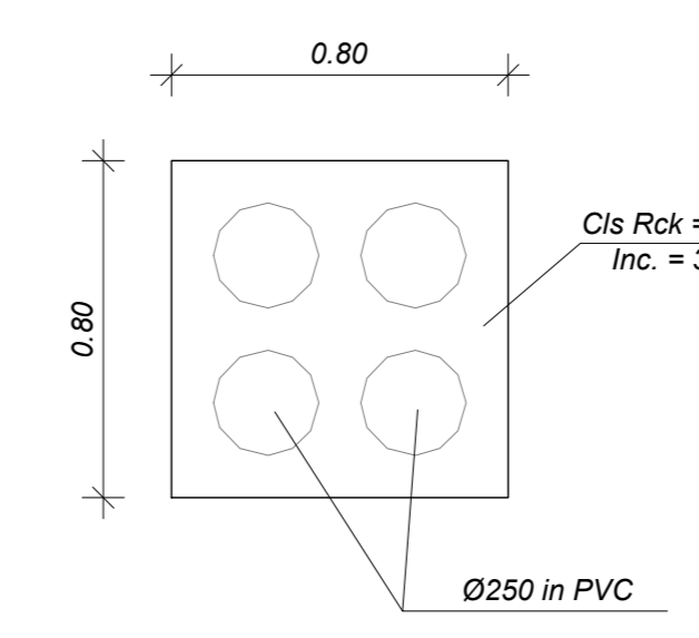
Dettaglio "3" - Canalizzazioni per alimentazione elettrica linea
