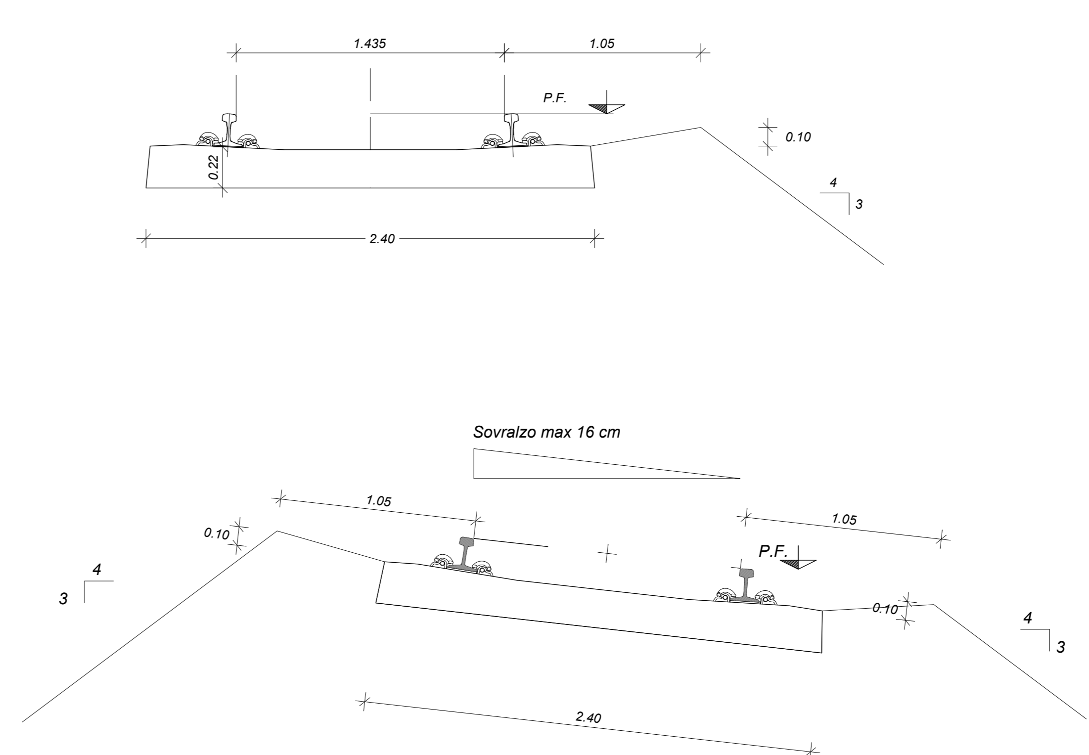
Dettaglio "1" - Andamento traversa in rettilineo ed in curva
