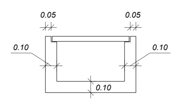
Dettaglio "4" - Canaletta idraulica al piede dell'opera di sostegno
