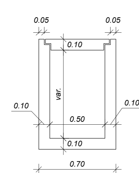
Dettaglio "2" - Canaletta idraulica
