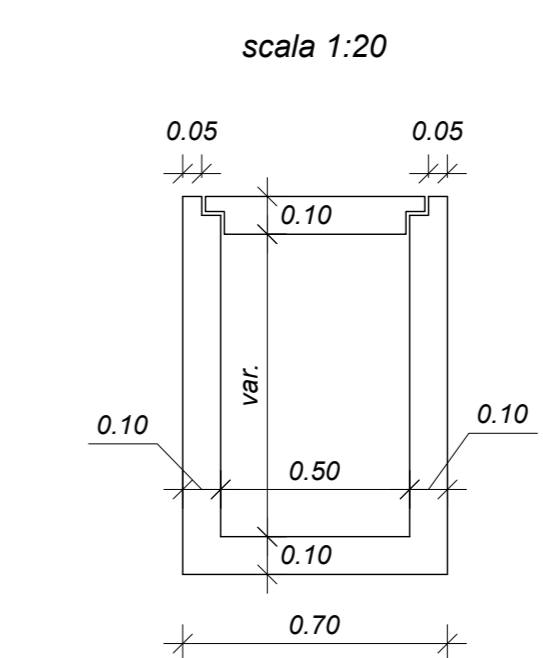
Dettaglio "2" - Canaletta idraulica
