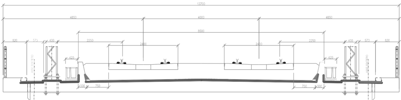
Fig. 35 – Sezione tipo ferroviaria ponte a doppio binario
