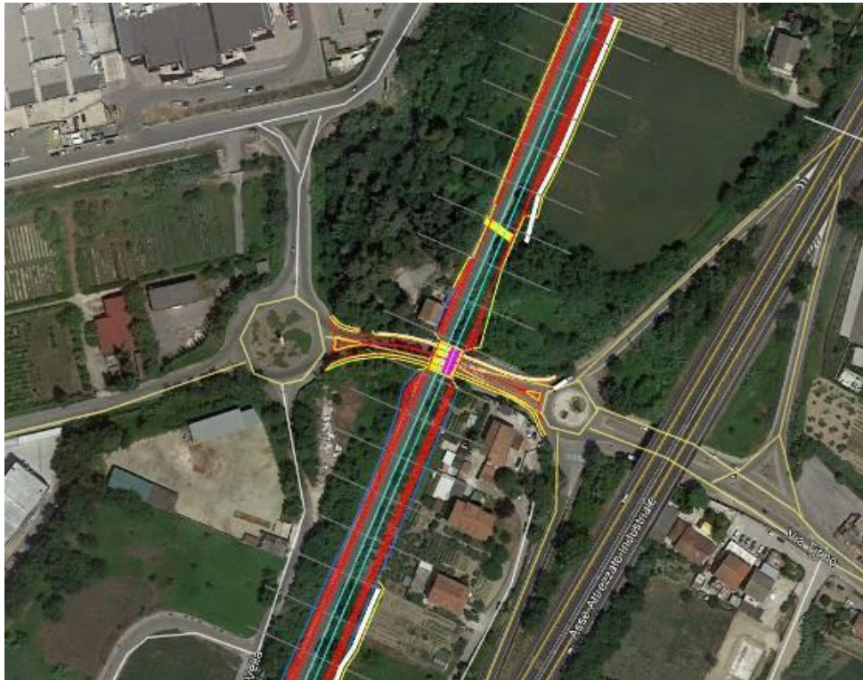
Fig. 45 – Viabilità stradale Via Tirino, sottovia al km 14+250.00 (NV34)
