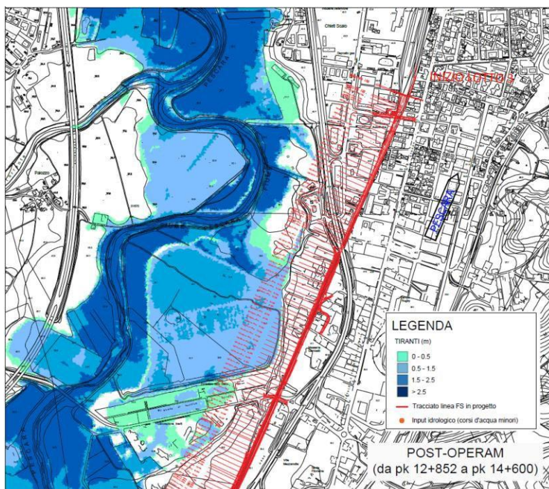
Fig. 25 – Modello numerico 2D: aree di esondazione Tr 300 anni del F. Pescara e dei due corsi d'acqua minori considerati, scenario post operam, pk 12+852 ÷ 14+600.
