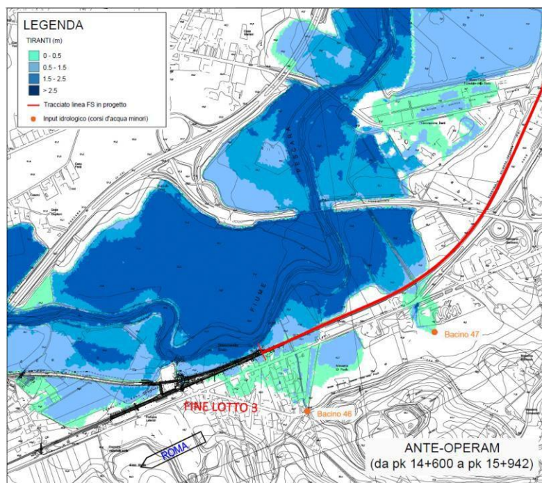
Fig. 20 – Modello numerico 2D: aree di esondazione Tr 200 anni del F. Pescara e dei due corsi d'acqua minori considerati, scenario ante operam, pk 14+600 ÷ 15+942.
