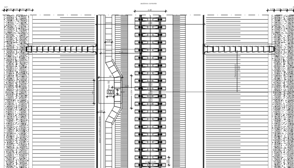
Fig. 31 – Stralcio planimetrico per sezione tipo ferroviaria in rilevato a singolo binario (piattaforma in retto) con H_{ril} \leq 6,00 m
