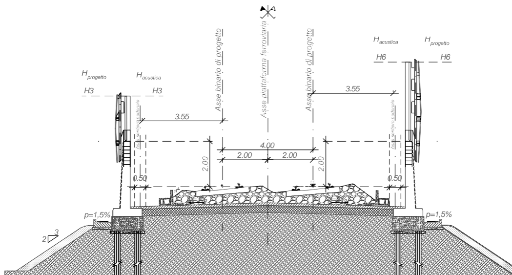
Fig. 51 – Sezione tipo tipologica BA "HS" rettificato con manufatto prefabbricato su rilevato
