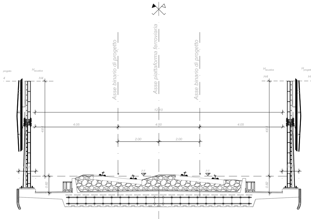
Fig. 53 – Sezione tipo tipologico BA “HS” rettificato su impalcato ferroviario
