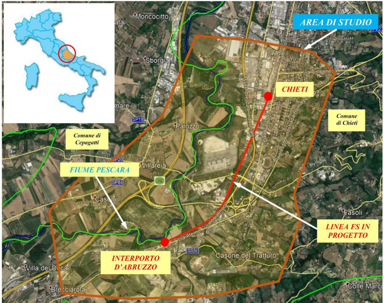
Fig. 16 – Inquadramento geografico della zona in esame con evidenziata la linea ferroviaria in affiancamento al F. Pescara.
