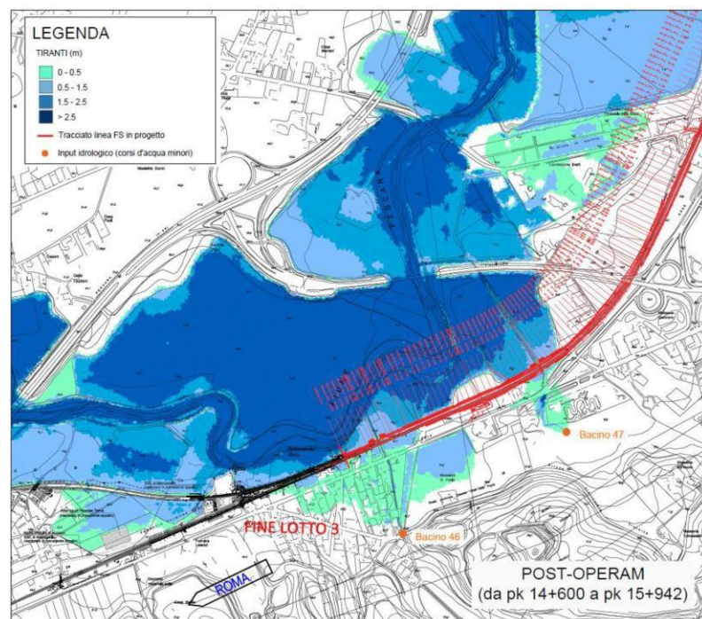
Fig. 22 – Modello numerico 2D: aree di esondazione Tr 200 anni del F. Pescara e dei due corsi d'acqua minori considerati, scenario post operam, pk 14+600 ÷ 15+942.
