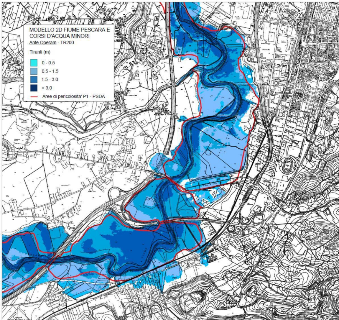
Fig. 18 – Modello idraulico 2D: aree di esondazione (Tr 200 anni) del F. Pescara e dei cinque corsi d'acqua minori considerati; confronto con le aree di pericolosità idraulica P1 del PSDA (zona Chieti).
