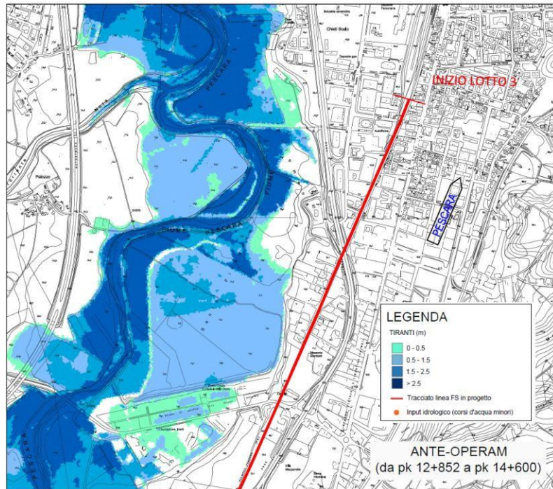
Fig. 19 – Modello numerico 2D: aree di esondazione Tr 200 anni del F. Pescara e dei due corsi d'acqua minori considerati, scenario ante operam, pk 12+852 ÷ 14+600.
