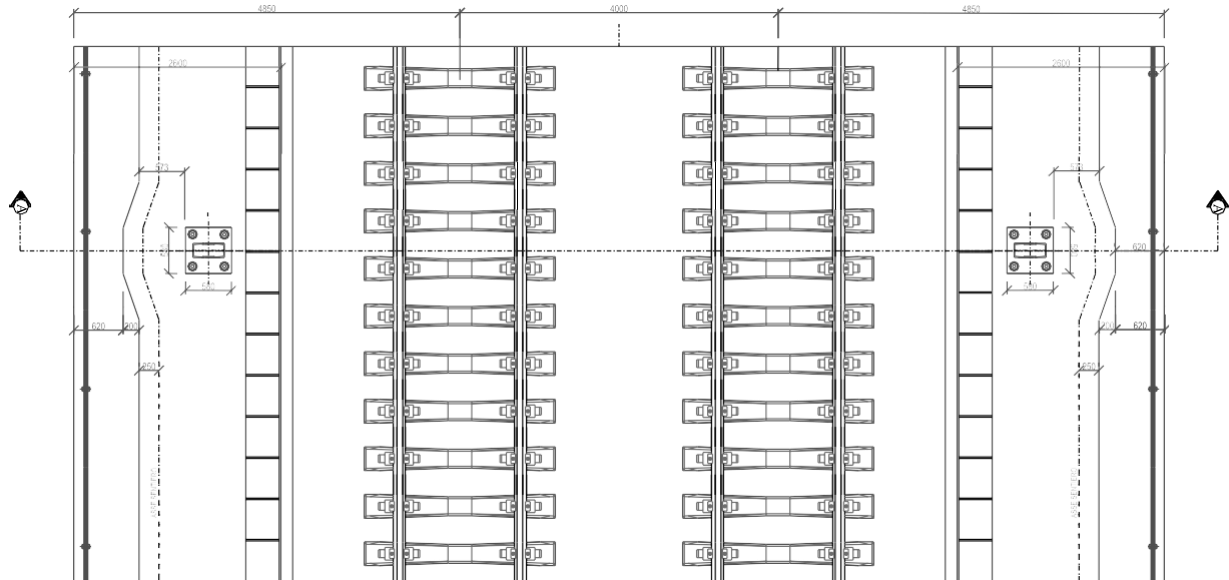
Fig. 33 – Stralcio planimetrico sezione tipo ferroviaria in viadotto a doppio binario
