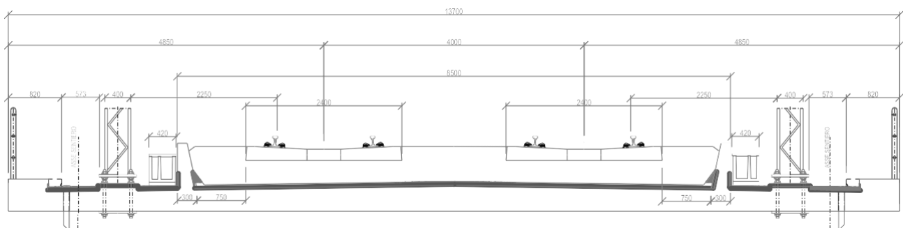
Fig. 32 – Sezione tipo ferroviaria in viadotto a doppio binario
