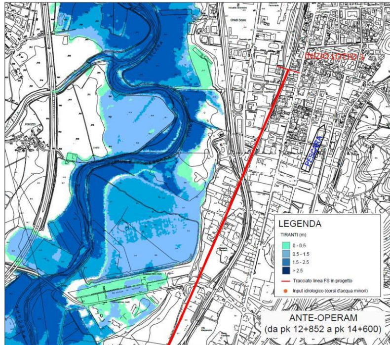
Fig. 23 – Modello numerico 2D: aree di esondazione Tr 300 anni del F. Pescara e dei due corsi d'acqua minori considerati, scenario ante operam, pk 12+852 ÷ 14+600.
