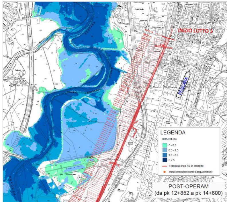
Fig. 21 – Modello numerico 2D: aree di esondazione Tr 200 anni del F. Pescara e dei due corsi d'acqua minori considerati, scenario post operam, pk 12+852 ÷ 14+600.
