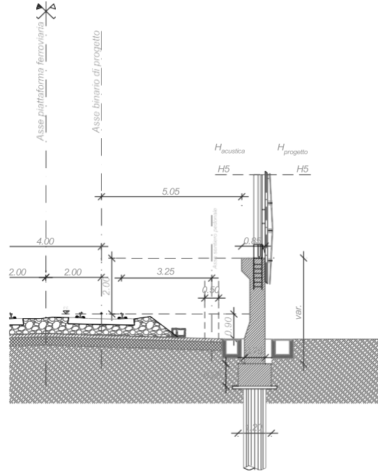
Fig. 52 – Sezione tipo tipologico BA “HS” rettificato senza manufatto prefabbricato fondato su OdS
