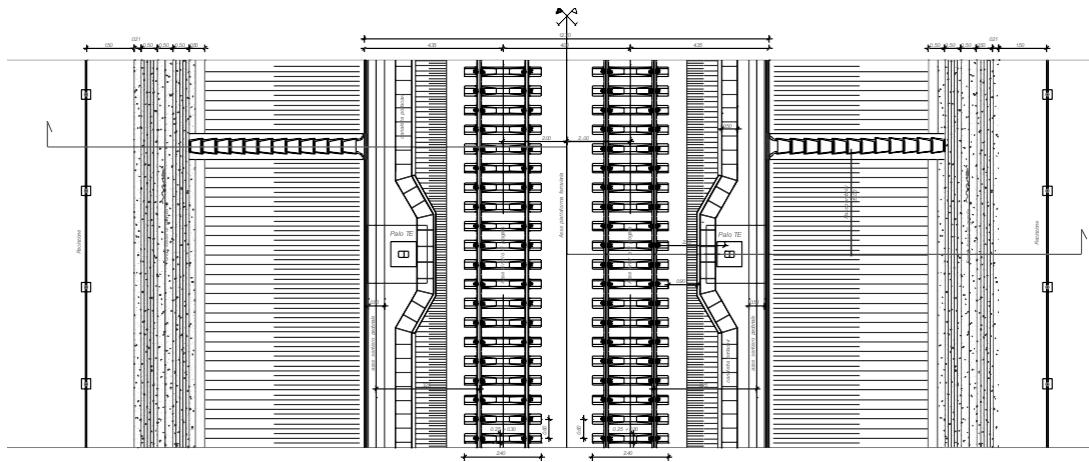
Fig. 28 – Stralcio planimetrico per sezione tipo ferroviaria in rilevato a doppio binario (piattaforma in retto) con H_{rl} \leq 6,00 m
