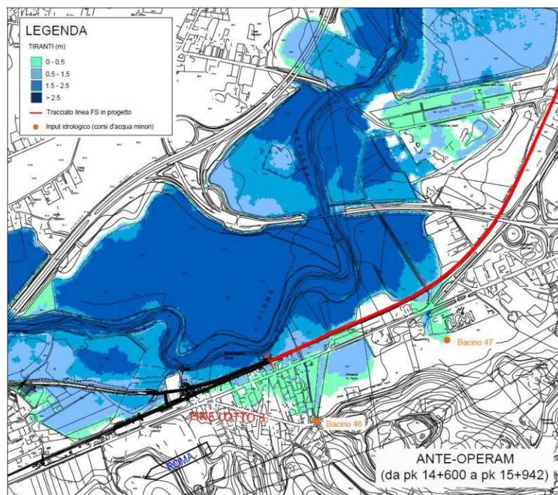
Fig. 24 – Modello numerico 2D: aree di esondazione Tr 300 anni del F. Pescara e dei due corsi d'acqua minori considerati, scenario ante operam, pk 14+600 ÷ 15+942.
