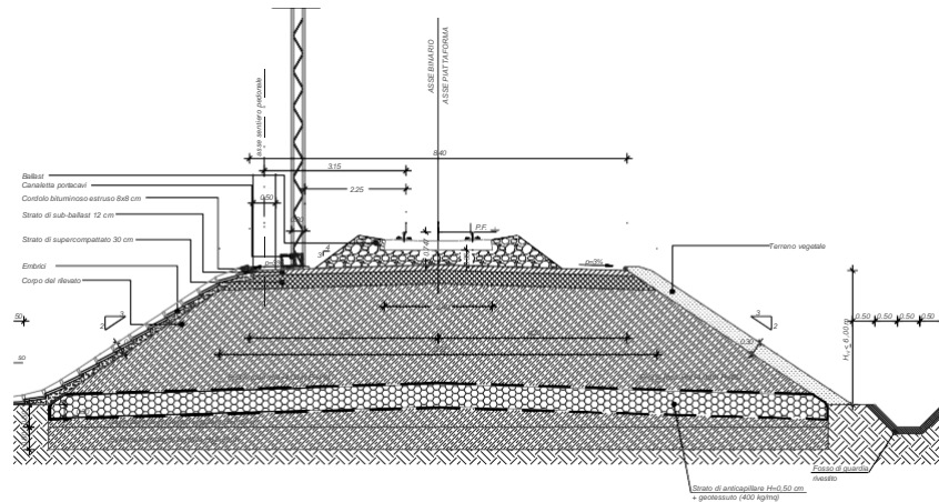
Fig. 30 – Sezione tipo ferroviaria in rilevato a singolo binario (piattaforma in retto) con H_{ril} \leq 6,00 m
