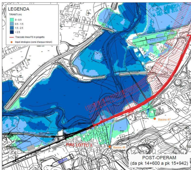
Fig. 26 – Modello numerico 2D: aree di esondazione Tr 300 anni del F. Pescara e dei due corsi d'acqua minori considerati, scenario post operam, pk 14+600 ÷ 15+942.
