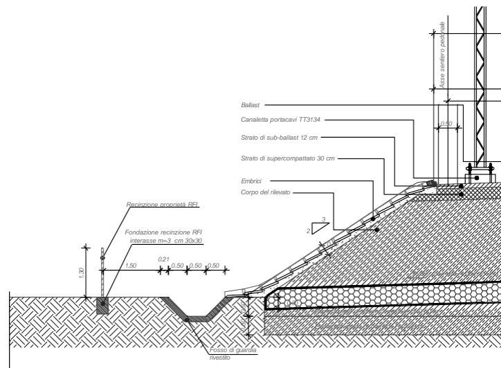
Fig. 29 – Dettaglio alla base del rilevato ferroviario
