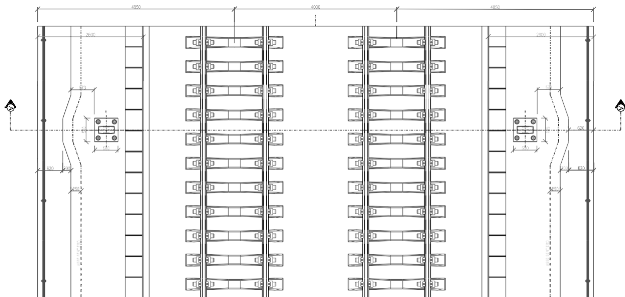
Fig. 36 – Stralcio planimetrico sezione tipo ferroviaria ponte a doppio binario
