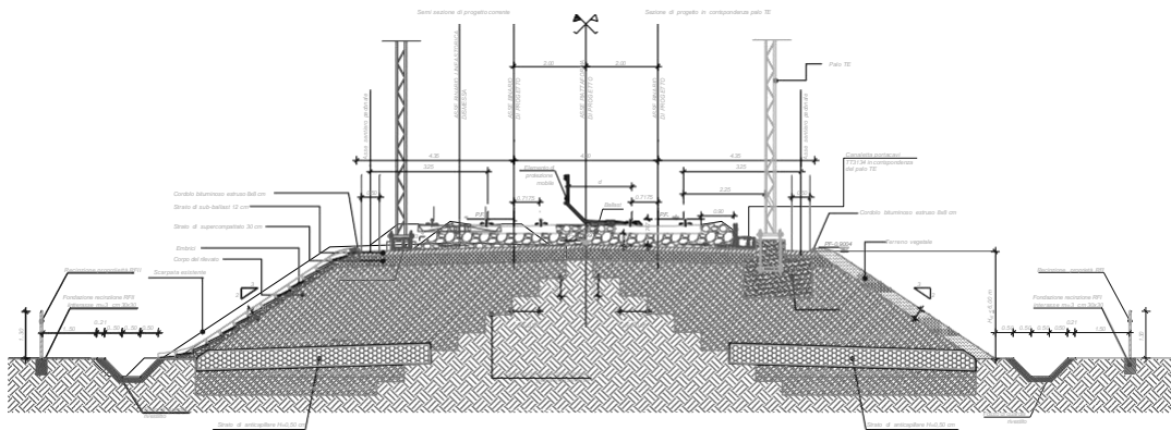
Fig. 27 – Sezione tipo ferroviaria in rilevato a doppio binario (piattaforma in retto) con H_{ri} \leq 6,00 m
