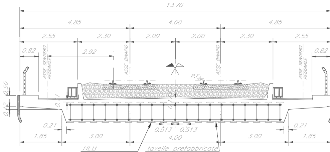
Fig. 37 – Sezione tipo ferroviaria impalcato a travi incorporate a DB
