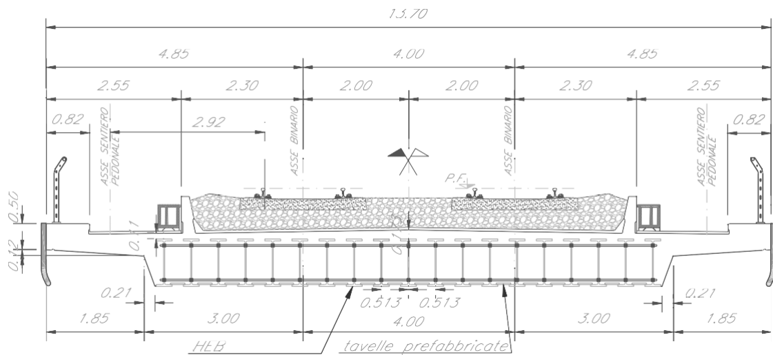
Fig. 34 – Sezione tipo ferroviaria impalcato a travi incorporate a DB
