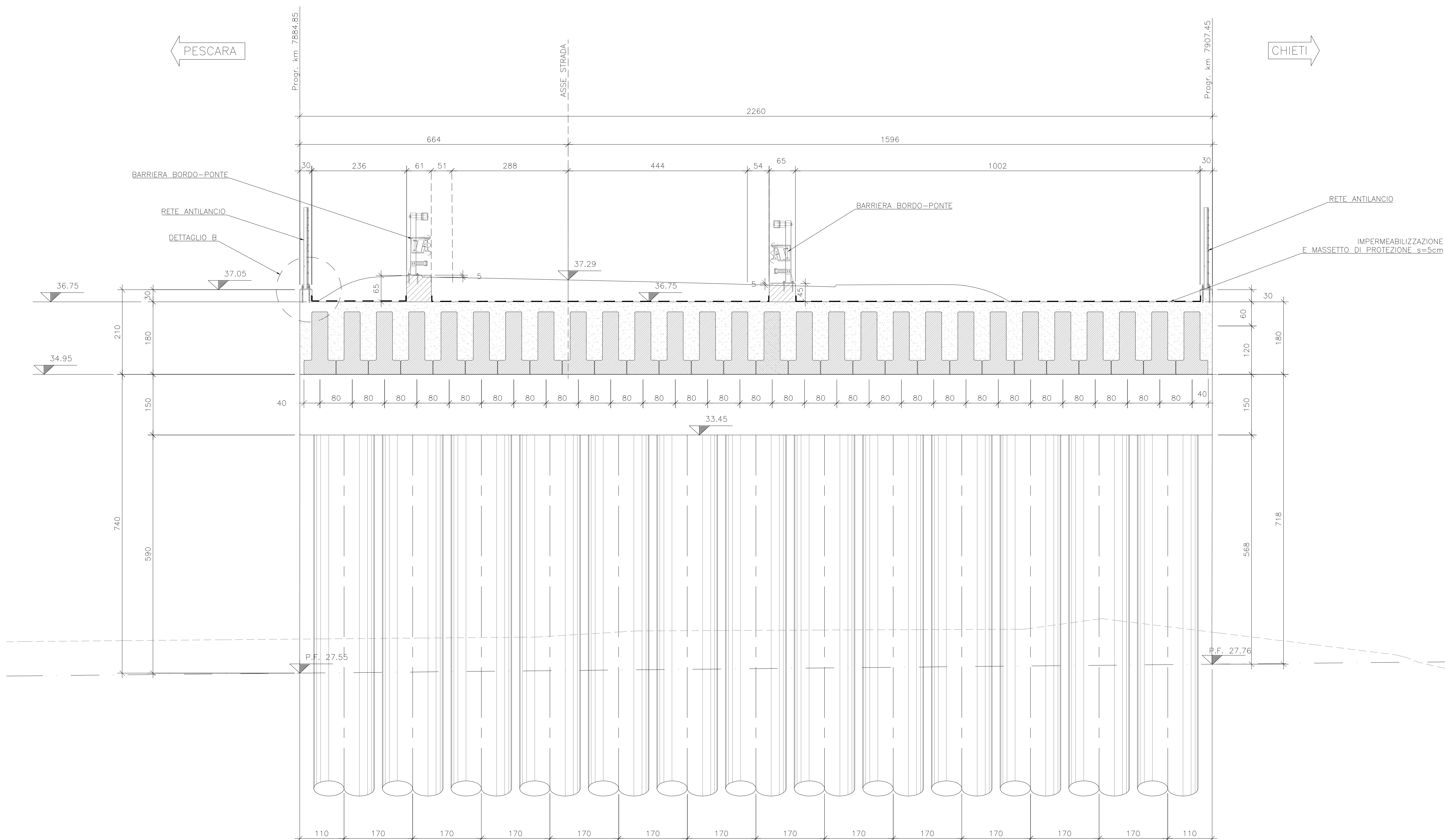
SEZIONE I-I IN ASSE BINARIO PARI Scala 1:50
