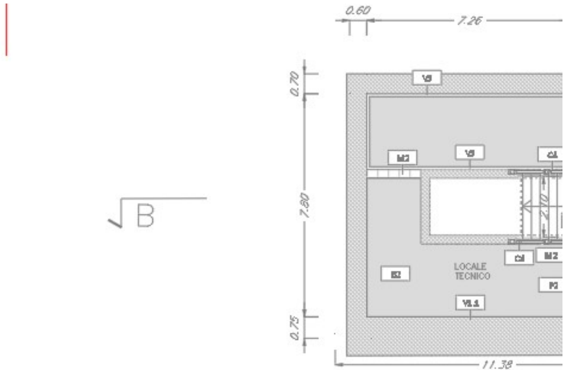
Figura 3. Pianta sottopasso
