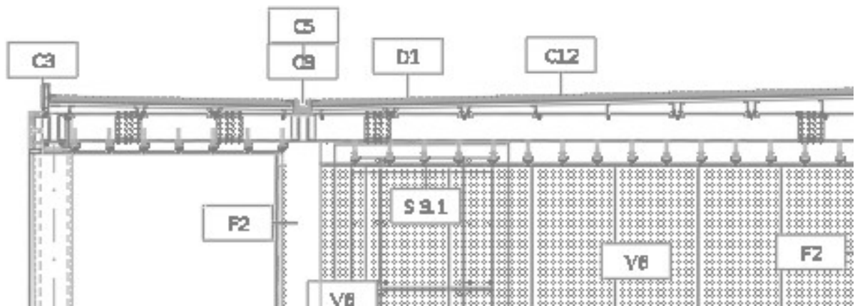
Figura 4. Sezione sottopasso
