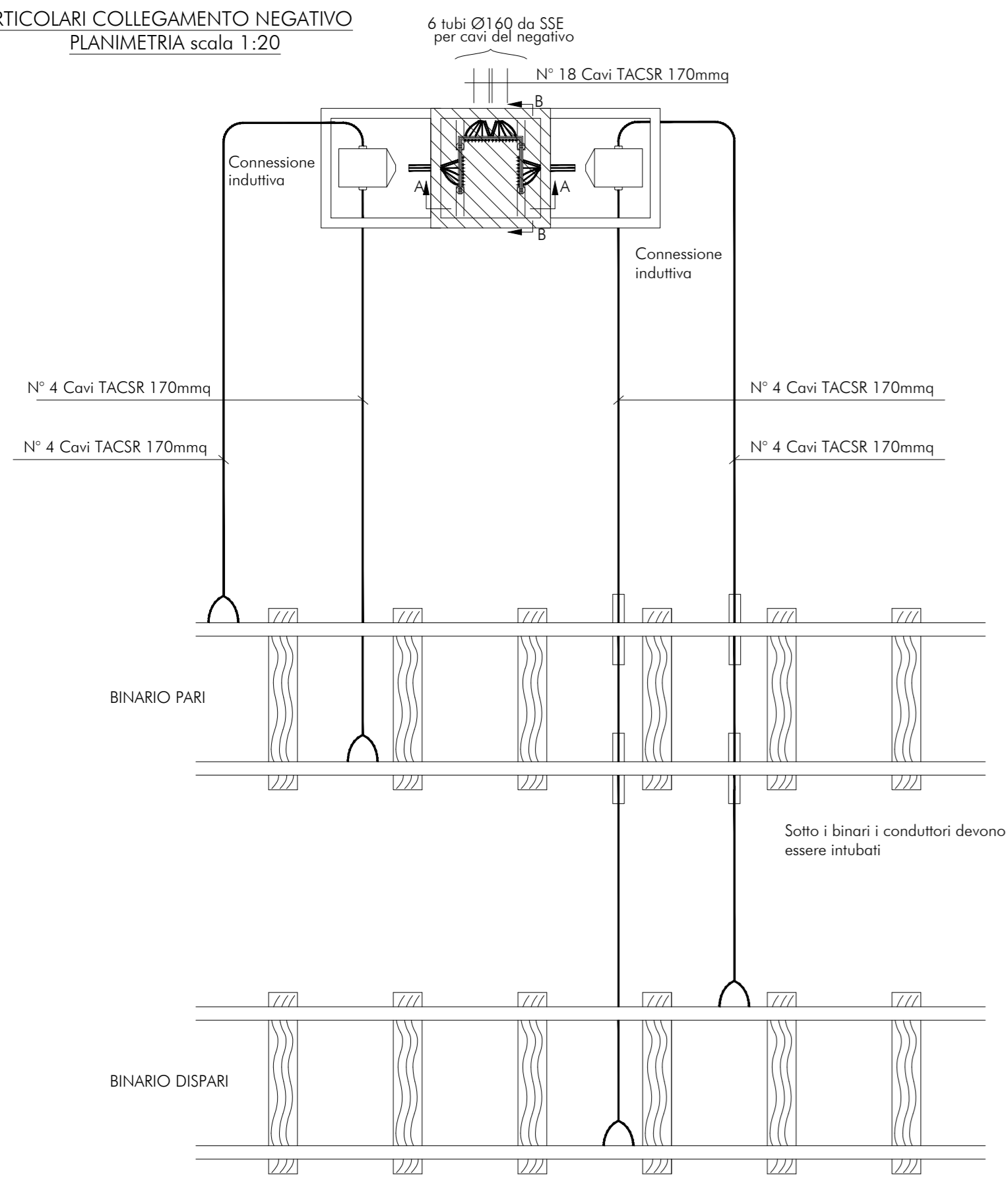
PARTICOLARI - CONNESSIONE AL BINARIO
