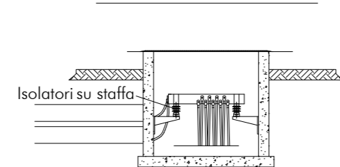
SEZIONE B-B scala 1:20
