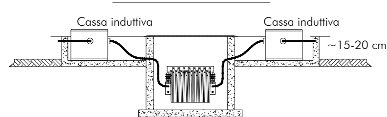
SEZIONE A-A scala 1:20
