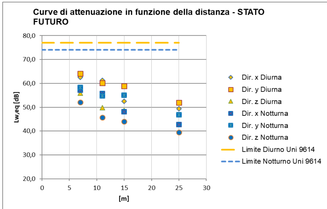
Figura 5 – Curve di attenuazione in funzione della distanza relativa al traffico ferroviario di progetto – Treni Totali Regionali + Mercı
