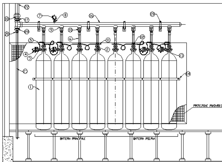
Figura 1 – Batterie di bombole
