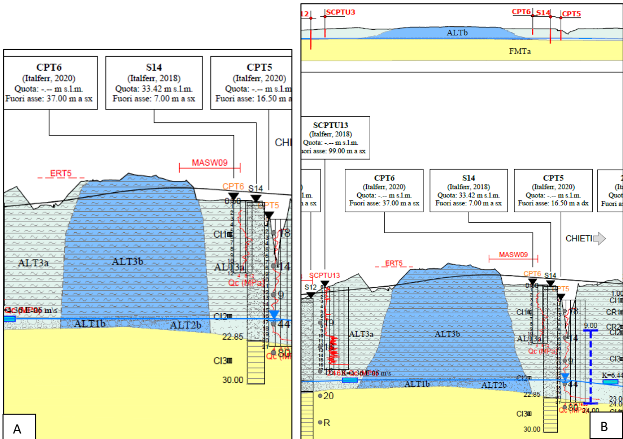
Figura 1. Stralcio del profilo geologico tra le pk 8+400 e pk 8+750 (A) IA4S 02 D69 N5GE0001001C, consegna al CS CSLLP a giugno 2023; Stralcio del profilo geologico (B) IA4S 02 D69 N5GE0001001D, consegna al CS CSLLP a settembre 2023 con aggiunta del profilo in scala verticale non deformata.
